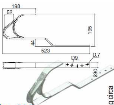
Art. 399 Gancio sottotegola Under roof tile hook
